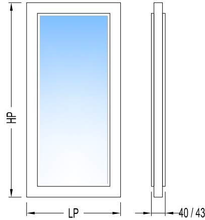
PANNEAU PORTE:
